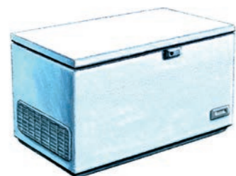
0404 Congélateur 600 L 220 V / 16A monophasé - 290 W. Pouvoir de congélation : 30 Kg / 24 h. Ext. L 165 ; P 81 ; H 89 cm. 75 Kg
