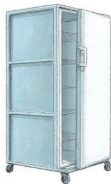
0684 Réfrigérateur 500 litres : 220 V / 16A 150 W. Ext. : L 75 ; l 70 ; H 151 cm. 75 Kg. Livré avec 5 grilles 68 x 52 cm. Ext. : L 80 ; l 80 ; H 180 cm.
