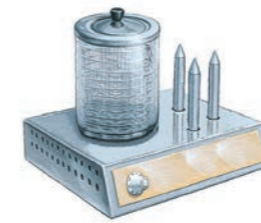
0419 Hot-dogger 220 V / 16 A monophasé - 650 W 1 couvercle, 1 manchon Ø 20 cm, 1 grille Ø 17,5 cm, 1 socle chauffant avec bac à eau. Ext. : L 45 ; I 29 ; H 42 cm. 13 Kg
